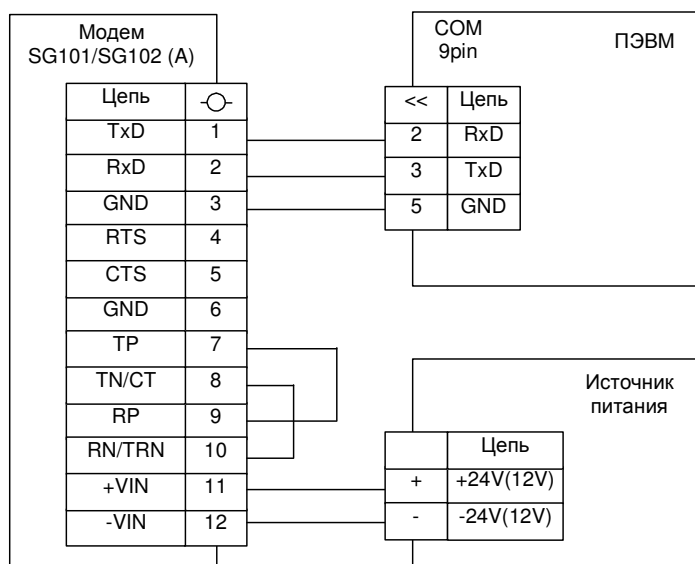
Рисунок 31 – Схема проверки функционирования модема исполнений 1 и 2 (вариант А – см. 5.11.2)
