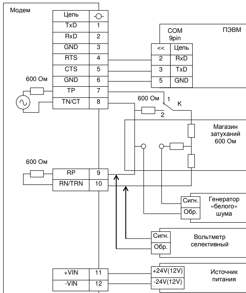
Рисунок 36 – Схема испытаний модема
