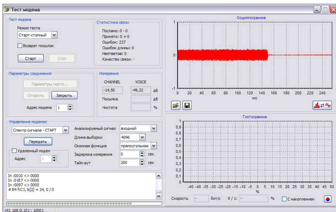
Рисунок 23 – Представление полученных данных (установленной выборки) на временной оси (осциллограмма сигнала)
