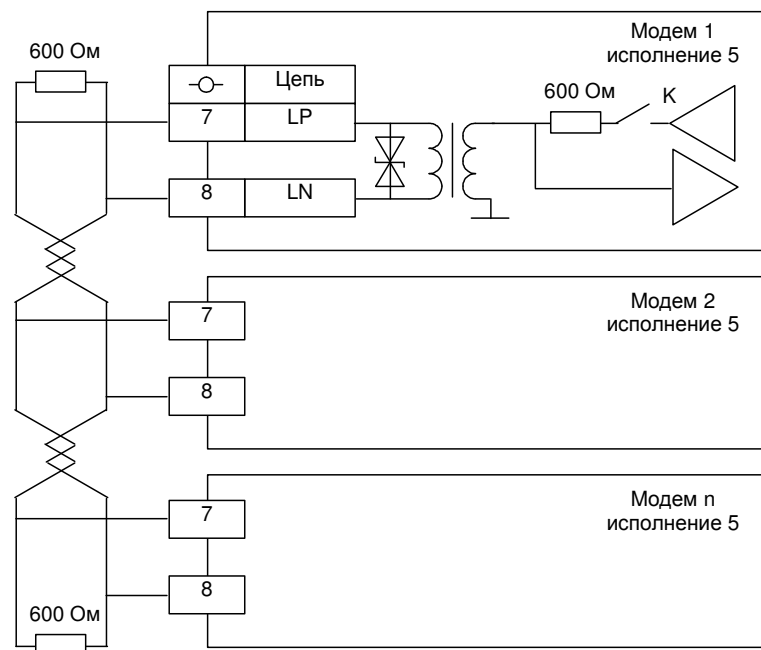
Рисунок 7 – Схема линейного узла стыка С1-ТЧ модема исполнения 5 и пример подключения n модемов к кабельной двухпроводной линии
