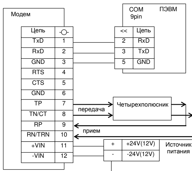
Рисунок 22 – Схема подключения четырехполюсника к модему для измерения АЧХ
