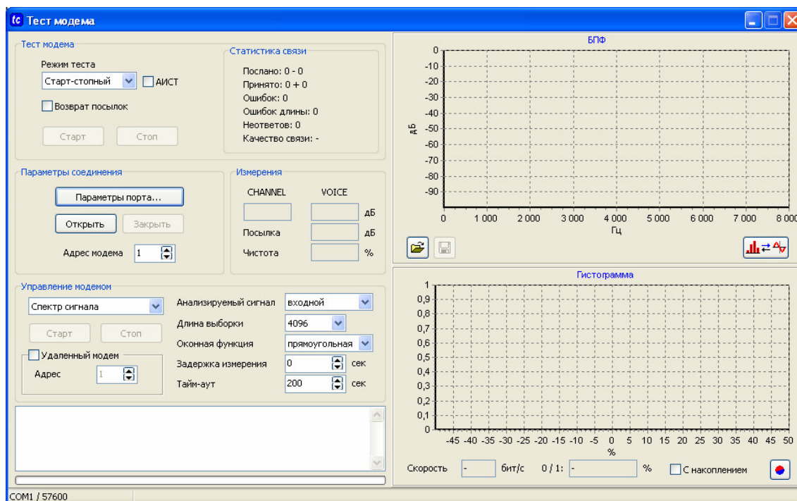
Рисунок 19 – Установка параметров измерительной процедуры модема
