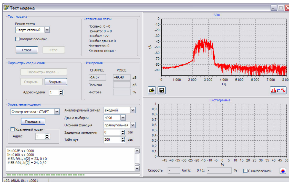
Рисунок 20 – Ход исполнения измерительной процедуры модема – спектр сигнала, и представление полученных данных на частотной оси (спектрограмма)
