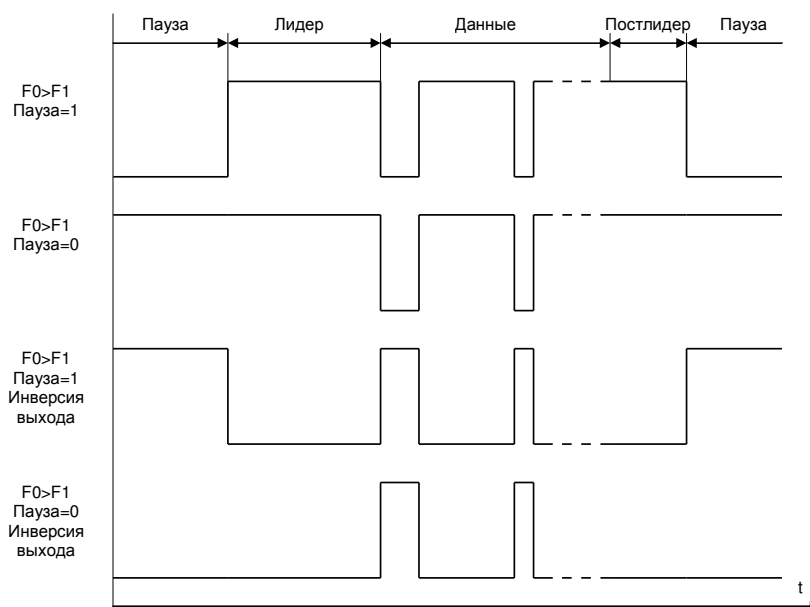
Рисунок 40 – Временные диаграммы сигнала на выходе RTS в режиме прямой передачи данных
