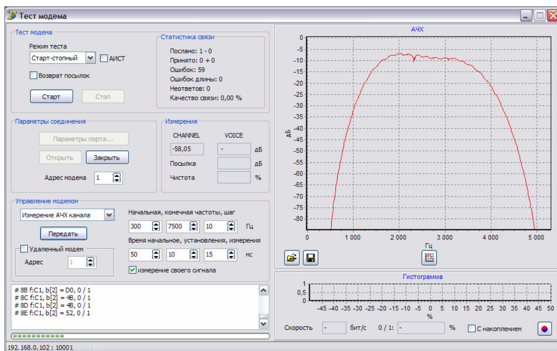
Рисунок 21 – Ход выполнения измерительной процедуры модема – измерение АЧХ тракта выход-вход, и представление полученных данных на частотной оси
