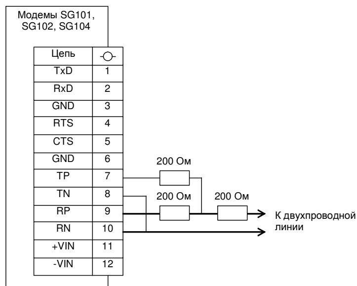
Рисунок 41 – Схема подключения четырехпроводного модема (исполнения 1, 2 и 4) к двухпроводной линии связи
