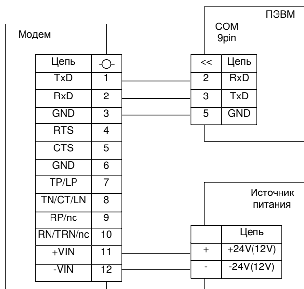
Рисунок 8 – Схема подключения модема для параметризации и записи FLASH-памяти
