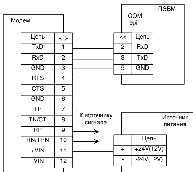
Рисунок 25 – Схема подключения модема для записи сигнала в файл
