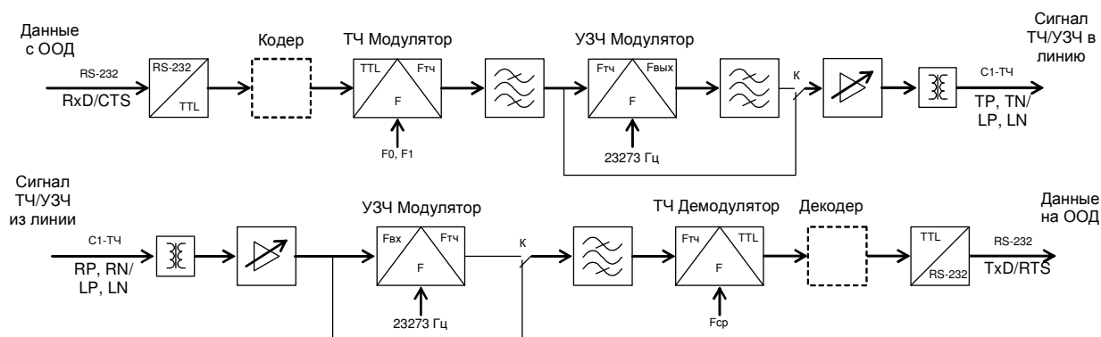
Рисунок 2 – Схема функциональная модема
