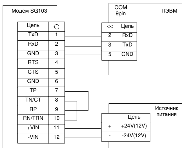
Рисунок 33 – Схема проверки функционирования модема исполнения 3
