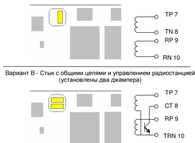
Рисунок 37 – Установка джамперов линейного узла для исполнения 2
