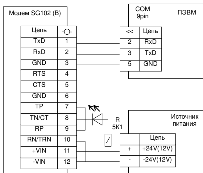
Рисунок 32 – Схема проверки функционирования модема исполнения 2 (вариант В – см. 5.11.2)
