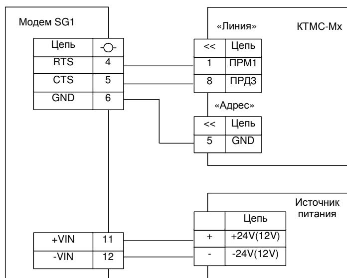
Рисунок 38 – Схема подключения модема к контроллеру КТМС-Мх
