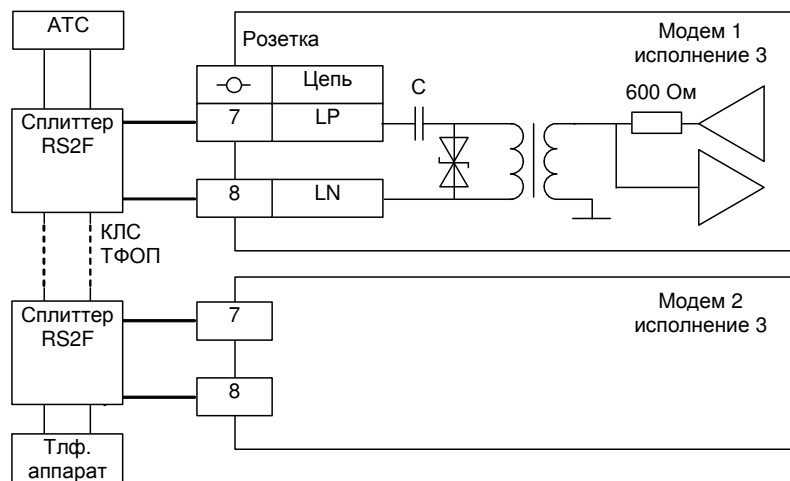
Рисунок 6 – Схема линейного узла стыка С1-ТЧ модема исполнения 3 и пример подключения двух модемов к кабельной линии ТФОП
